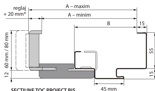
SECȚIUNE TOC PROIECT BIS
