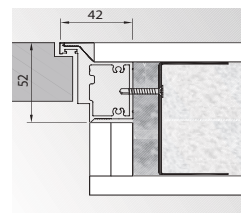
fără falț (deschidere spre exterior)
