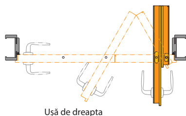
Modul de deschidere* (vedere de sus)
