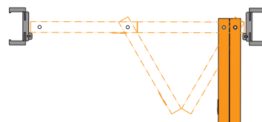
Modul de deschidere* (vedere de sus)
