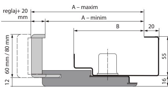
SECȚIUNE TOC PROIECT PREMIUM
